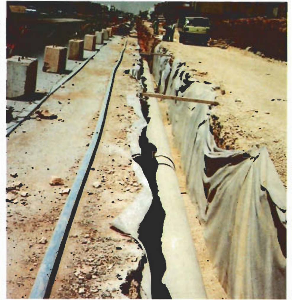
نظام صرف المياه الأرضية بالمريجة الغربية
